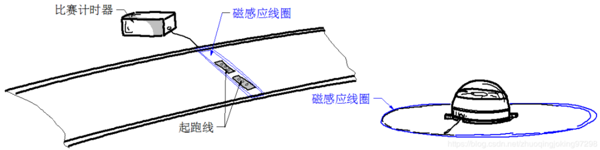
基于磁感应的比赛计时系统
